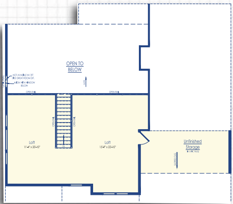
Optional Loft Elevation F
