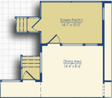
Optional Screen Porch I
