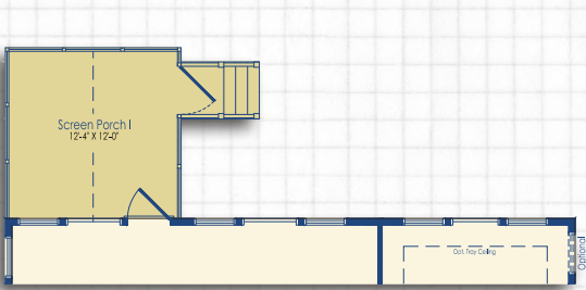
Optional Screen Porch I
