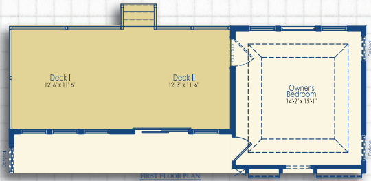
Optional Deck I & II
