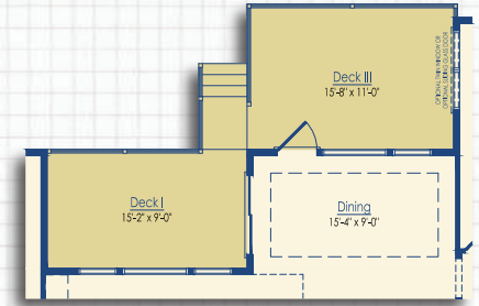
Optional Deck I & Optional Deck III
