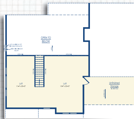
Optional Loft Elevation F
