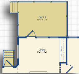
Optional Deck II
